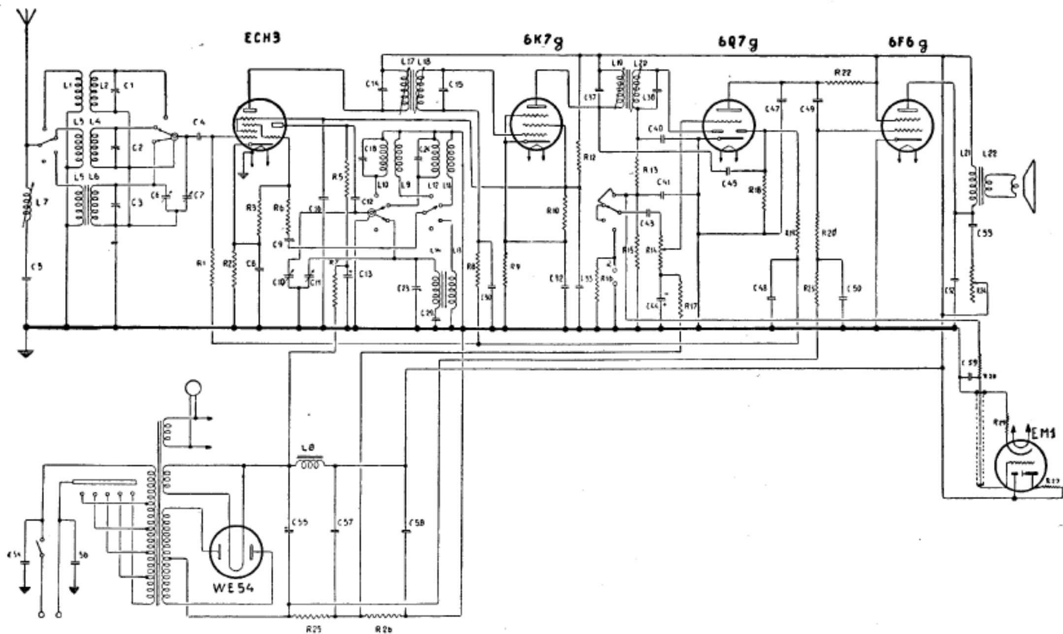
Fig. 97. - Ricevitore supereterodina a 5 valvole e 3 gamme d'onda. (C. G. E., mod. 1332 - mod. 1331 differisce solo per l'assenza della EMI, indicatrice di sintonia).
